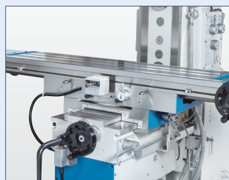
Der Frästisch verfügt über eine große Aufspannfläche und kann in Längsrichtung geschwenkt werden
