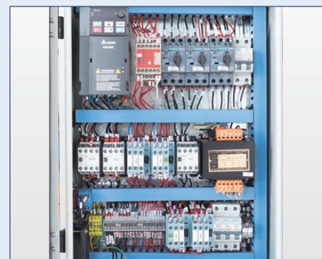
Hochwertige Komponenten sichern die Zuverlässigkeit u. Leistungsfähigkeit der Fräsmaschine
