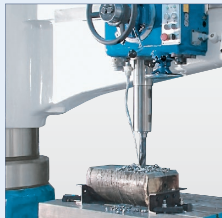
Eine einstellbare Überlastungskupplung schützt Werkstück und Maschine vor Beschädigungen
