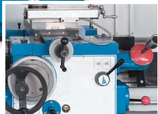
Die Nebenzeiten reduzierend, kann der Support in Längs- und Querrichtung motorisch im Eilgang verfahren werden
