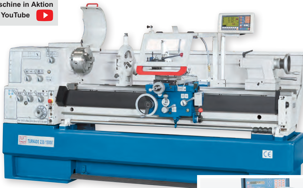
Abb. Turnado 230/1500 V mit 3-Achs-Positionsanzeige und stufenloser Drehzahlverstellung
