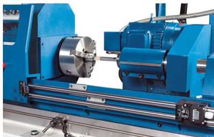
La poupée de rectification peut être pivotée à 180° pour passer de la rectification intérieure à la rectification extérieure
