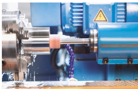
La rectification intérieure est possible jusqu'à une profondeur de 125 mm
