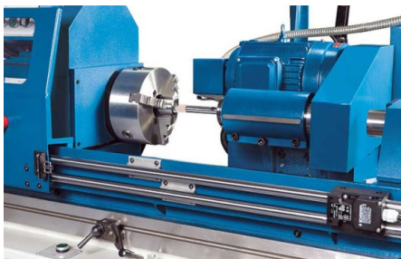
Brousící vřeteník je možné otočit pro změnu vnitřního na vnější broušení o 180°
