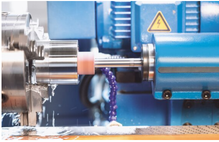
Innenschleifen ist bis zu einer Tiefe von 125 mm möglich
