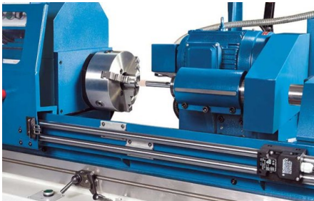
Schleifspindelstock kann zum Wechseln vom Innen- zum Außenschleifen um 180° gedreht werden
