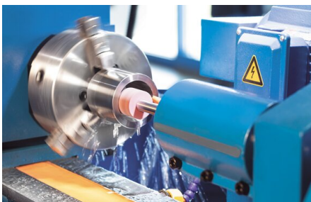
Der maximale Innenschleifdurchmesser beträgt 100 mm
