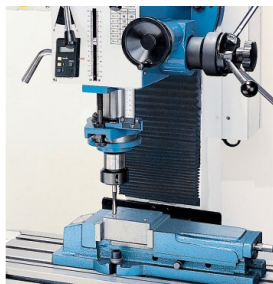
Vrtání závitů
