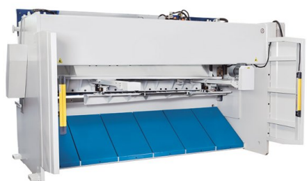
Sistem cu barieră fotoelectrică în partea din spate pentru un plus de protecție
