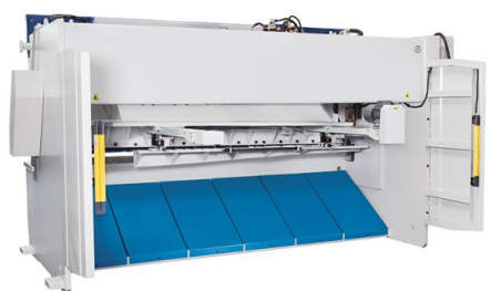
Systém světelné závoří v zadní části zajišťuje vyšší ochranu
