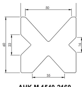
Maszyna jest standardowo dostarczana z europejskim narzędziem dolnym 4V
