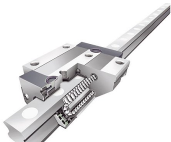
Guidages à rouleaux de haute qualité
