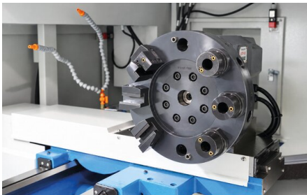
8-fach Werkzeugrevolver mit VDI 30
