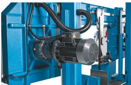
Motor de accionamiento principal potente, infinitamente variable
