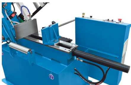
Fălciile de prindere pot fi rabatate manual până la 45°
