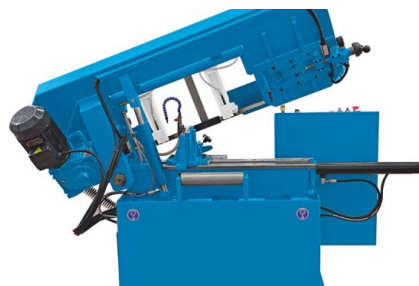
Motorul cu turații reglabile fără trepte își transmite puterea printr-un angrenaj de deviere proiectat pentru funcționarea continuă asupra roții de propulsie a mașinii
