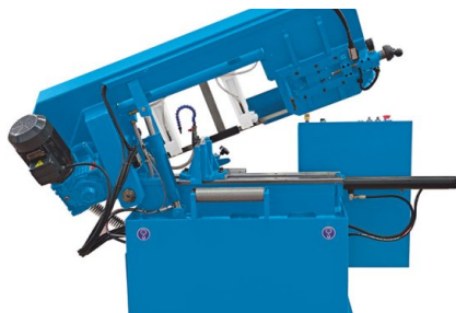
Motor s plynule regulovatelnými otáčkami přenáší svou sílu přes úhlovou převodovku, jež je dimenzována na trvalý provoz, na hnací kolo stroje
