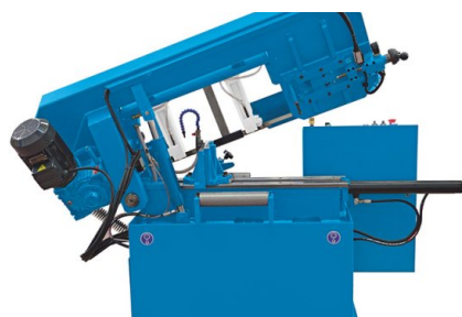
Silnik z płynnie regulowaną prędkością obrotową przenosi siłę przez przekładnię kierunkową przystosowaną do trybu ciągłego na koło napędowe maszyny
