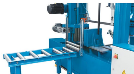
Rail stable d'acheminement à rouleaux et guidage de matière pour ensemble de pièces
