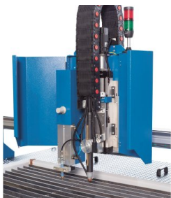
Rychlospojka pro řezací hlavu
