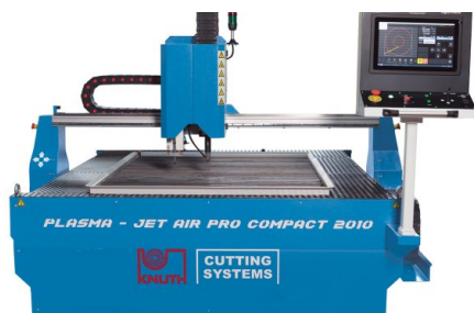
Jednodílná konstrukce s vedeními integrovanými do rámu stolu umožňuje přepravu zařízení ve smontovaném stavu a zaručuje rychlé a snadné uvedení do provozu
