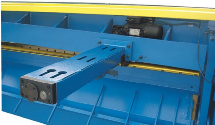
Der robuste Hinteranschlag ist dem Produktionsalltag gewachsen
