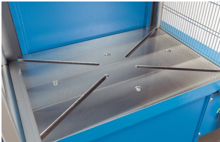
Des rainures alignées en diagonale facilitent le serrage centré des outils
