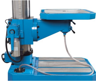
Motorische Höhenverstellung des Arbeitstisches
