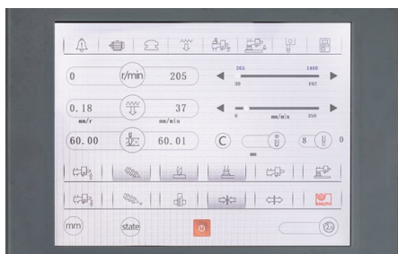
Avans pinolă cu reglare electronică cu ecran mare cu funcție de atingere
